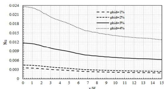
شکل ۱۵-ناسلت موضعی رژیم آشفته Re=1040 روی دیواره پایینی
