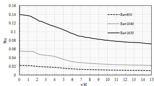
شکل ۱۳- ناسلت موضعی رژیم آشفته روی دیواره پایینی میکروکانال در پشت ریب با نسبت‌های دید و انسداد \frac{l}{d} = 9 و \frac{d}{H} = 0.4 و کسر حجمی نانوذرات \phi = 1\% در آب
