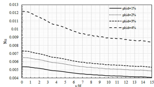
شکل ۱۴-ناسلت موضعی رژیم آرام Re=230 روی دیواره پایینی
