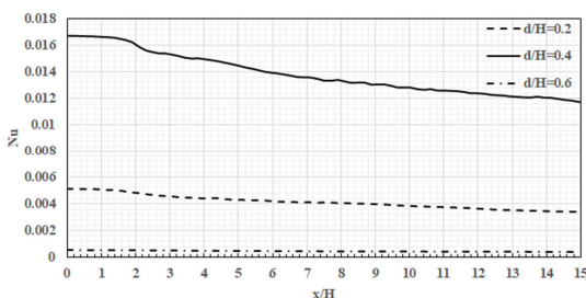
شکل ۱۶-تاثیر نسبت انسداد ریب بر انتقال گرما در رژیم جریان
