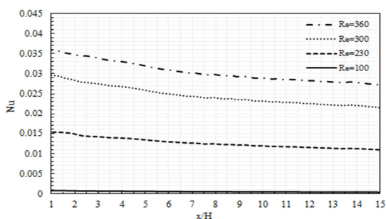
شکل ۱۲- ناسلت موضعی رژیم لایه‌ای روی دیواره پایینی میکروکانال در پشت ریب با نسبت‌های دید و انسداد \frac{l}{d} = 9 و \frac{d}{H} = 0.4 و کسر حجمی نانوذرات \phi = 1\% در آب
