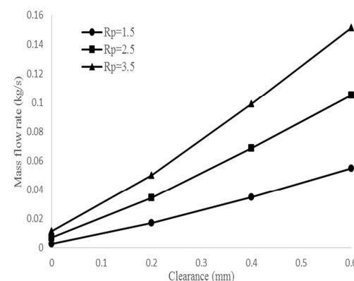
شکل ۱۴- تغییرات دبی جرمی هوا نسبت به لقی شعاعی رشته‌های براش سیل
