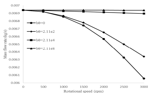
شکل ۱۶- تاثیر سرعت روتور بر دبی جرمی هوا ( \theta_0 = 0 )
