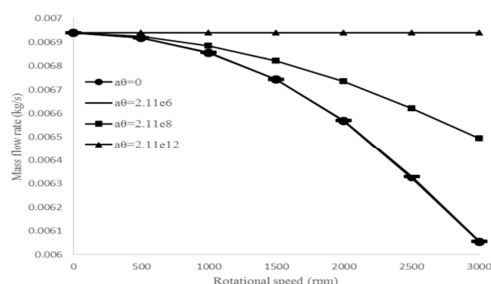
شکل ۱۵- تاثیر سرعت روتور بر دبی جرمی هوا ( \theta_0 = 0 )
