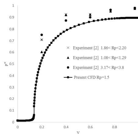
شکل ۶- مقایسه تغییرات فشار بی بعد در طول حلقه پشتی
