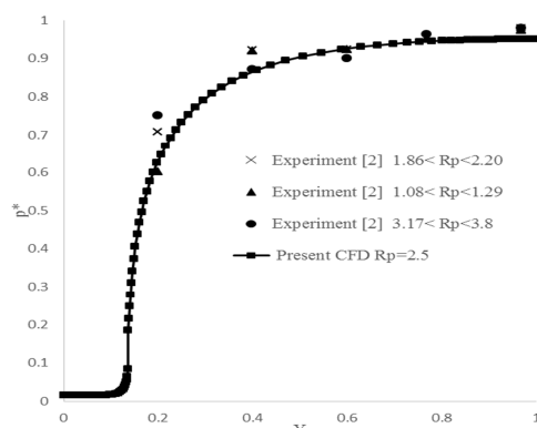
شکل ۷- مقایسه تغییرات فشار بی بعد در طول حلقه پشتی
