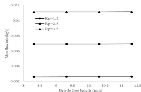
شکل ۱۰- تغییرات دبی جرمی هوا نسبت به طول آزاد رشته‌های براش سیل
