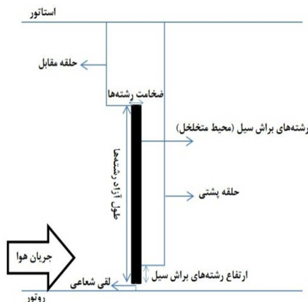
شکل ۱- ساختمان یک براش سیل
