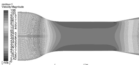
شکل ۴- کانتهورهای سرعت جریان در مجموعه نازل و اتاق آزمون و دیفیوزر
