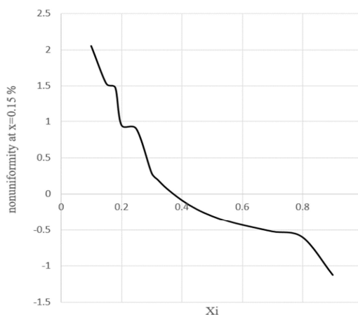
شکل ۱۱- غیریکنواختی بر روی خط طولی میانه گذرنده از مرکز اتاق آزمون در پروفیل‌های مختلف
