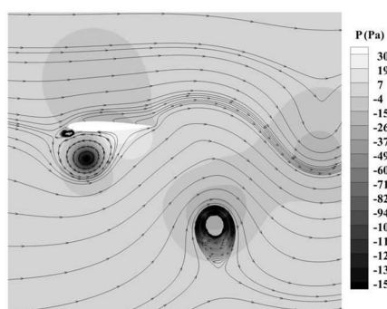
الف- بالاترین مکان نوسان ( t=T ) در حالت بدون پلازما
