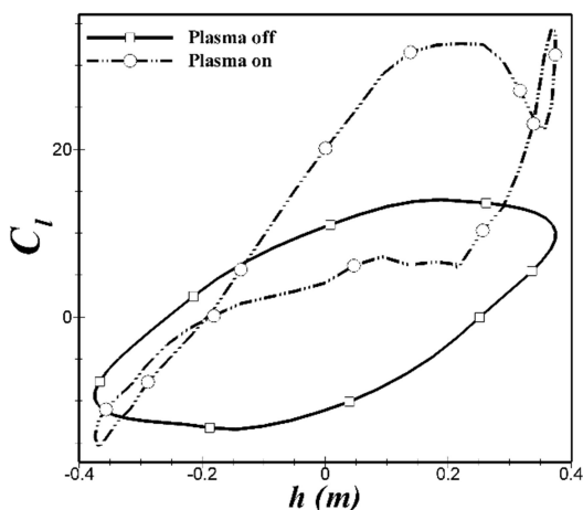
شکل ۱۰- مقایسه ضریب برآ برحسب دامنه نوسان با و بدون عملگر پلاسمایی در k=2/11
