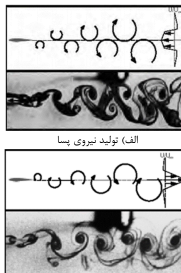
شکل ۱۱- ساختار گردابه ها درون دنباله [۲۰]
