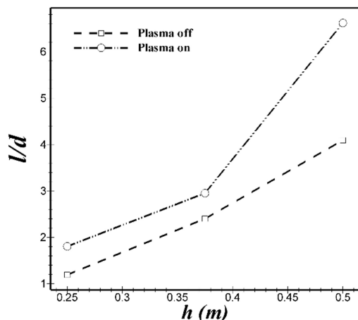
شکل ۱۸- بازده آیرودینامیکی متوسط برحسب دامنه نوسان در حضور و عدم حضور عملگر پلاسما
