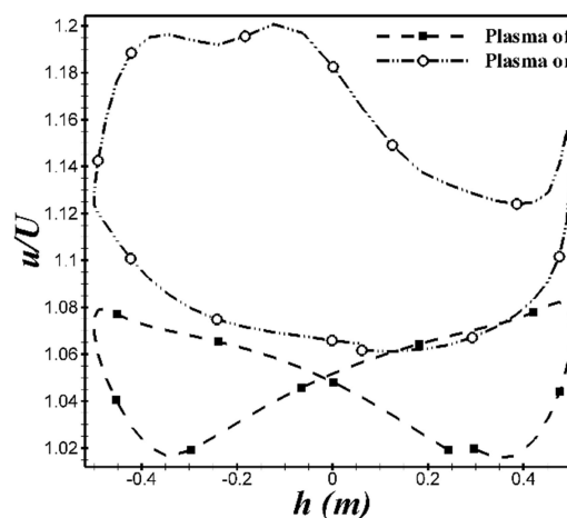
شکل ۱۵- حلقه هیستریسیس سرعت با و بدون عملکرد پلاسمایی، x/c=1
