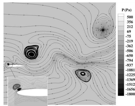
د- پایین ترین محل نوسان ( t = T/2 ) در حالت پلاسما روشن شکل ۱۶- کانتور فشار و خطوط جریان حول ایرفویل با نوسان انتقالی در حضور و عدم حضور عملگر پلاسمایی در h=0.5 c و k=2.11
