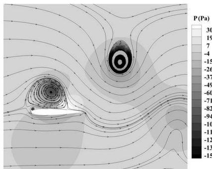
ب- پایین‌ترین مکان نوسان ( t=T/2 ) در حالت بدون پلازما
