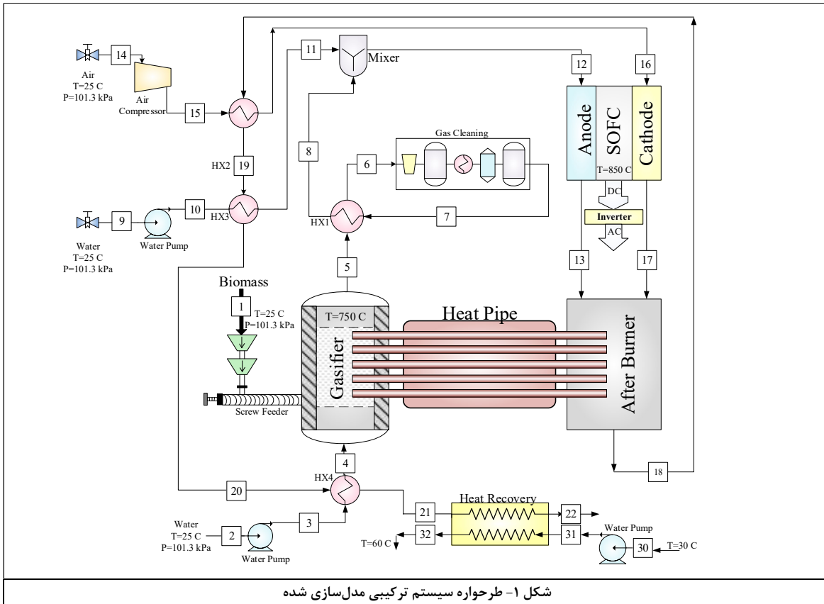
شکل ۱- طرحواره سیستم ترکیبی مدل‌سازی شده
