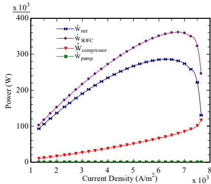
شکل ۸- تغییرات توان‌های سیستم با چگالی جریان
