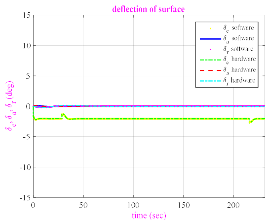
شکل ۱۶- انحراف سطوح کنترل پهپاد
