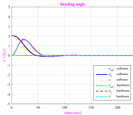
شکل ۱۱- تغییرات زاویه سمت
