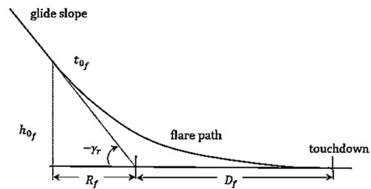
شکل ۵- هندسه مسیر فلر
