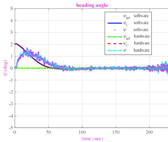
شکل ۲۱- تغییرات زاویه سمت در حضور اغتشاشات باد
