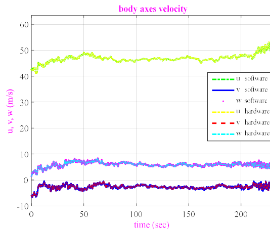
شکل ۲۳- سرعت های خطی در حضور اغتشاشات
