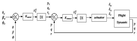
شکل 1- دیاگرام بلوکی حلقه آهسته همراه با حلقه سریع
