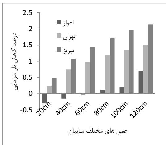
شکل ۴- کاهش مصرف انرژی با استفاده از سایبان
