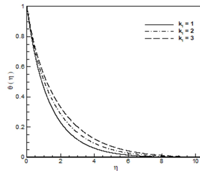
شکل ۴- تغییرات پارامتر k_1 بر روی دمای بی‌بعد
