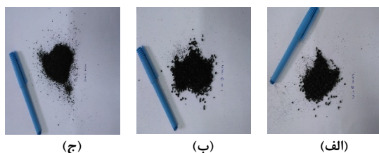
شکل ۲- ذرات لاستیک تایر ضایعاتی در اندازه (الف) 0-1 میلیمتر (ب) 1-3 میلیمتر (ج) 3-5 میلیمتر
