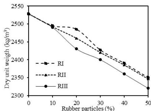
شکل ۹- چگالی بتن برحسب درصد ذرات لاستیک تاثیر ضایعاتی
