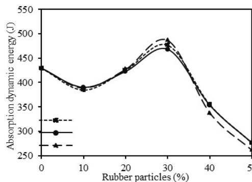
شکل ۱۹- میزان انرژی دینامیکی جذب شده بر حسب درصد ذرات لاستیک تایر ضایعاتی
