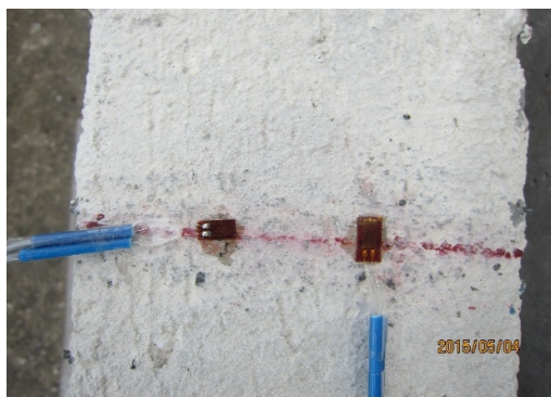
شکل ۱۴- کرنش سنج چسبیده بر سطح بتن حاوی ذرات لاستیک تایر ضایعاتی در فاصله ۱۰ سانتیمتری از تکیه گاه
