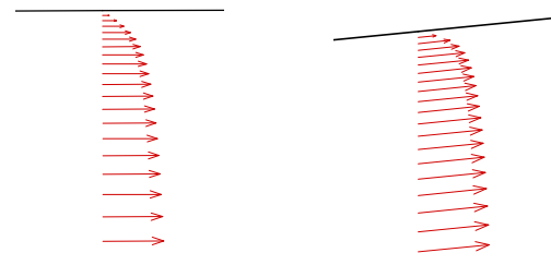
شکل ۲۴- بردارهای سرعت در نزدیک دیواره نازل مخروطی و منحنی‌دار
