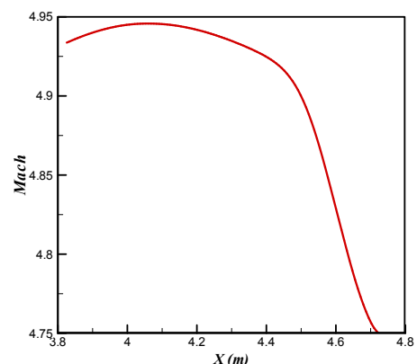
شکل ۲۳- نمودار عدد ماخ روی محور محفظه آزمون با نازل منحنی‌دار - با عدد ماخ ۵
