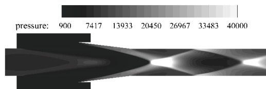
شکل ۲۷- کانطور فشار داخل محفظه آزمون و دیفیوزر
