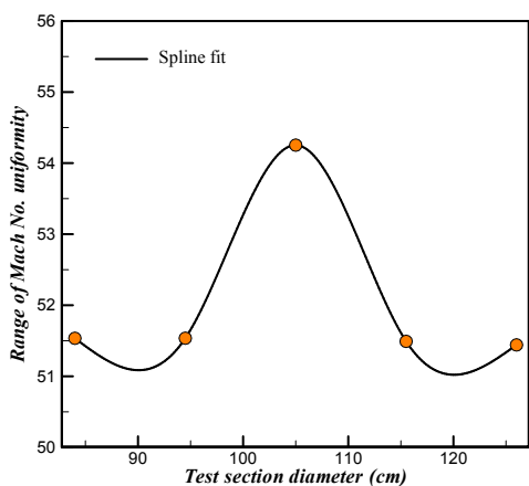
شکل ۱۷- محدوده یکنواختی عدد ماخ نسبت به تغییرات قطر محفظه آزمون- با عدد ۵ ماخ
