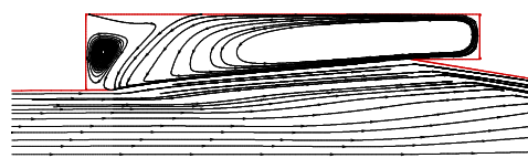
شکل ۱۹- خطوط جریان داخل محفظه آزمون-باعدد ماخ ۵
