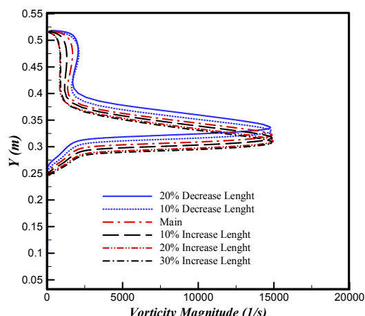
شکل ۱۳- توزیع گردابه برای مقاطع مختلف طول محور محفظه آزمون در x=440 cm
