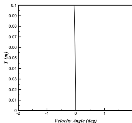
شکل ۲۰- میزان انحراف جریان نسبت به مقطعی در محدوده یکنواخت عدد ماخ - باعدد ماخ ۵
