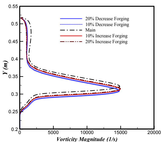
شکل ۱۶- توزیع گردابه برای فرورفتگی دیفیوزر داخل محفظه آزمون در x=440 cm - با عدد ماخ ۵
