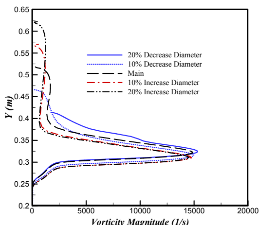
شکل ۱۸- توزیع ورتیسیتیته برای تغییرات قطر محفظه آزمون در x=440 cm - با عدد ۵ ماخ
