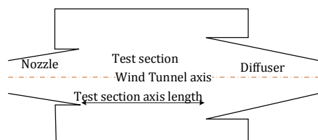
شکل ۸- نمایی از طول محور محفظه آزمون
