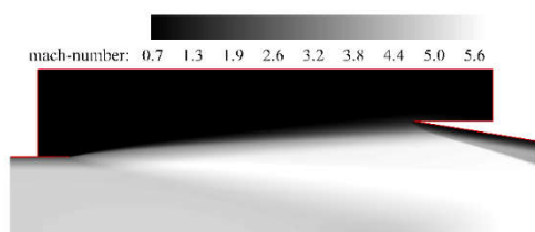
شکل ۲۵- کانتور عددماخ و خطوط جریان داخل محفظه آزمون
