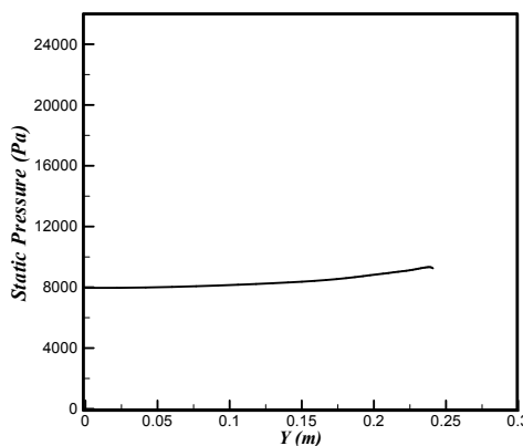
شکل ۲۰- منحنی تغییرات فشار استاتیکی در خروجی نازل- باعدد ماخ ۵
