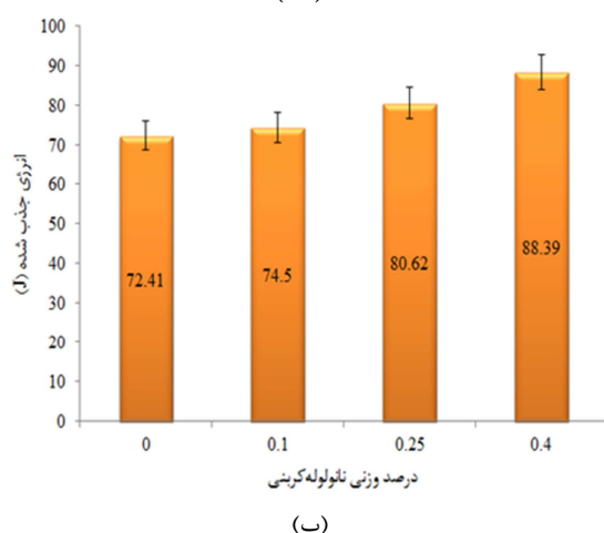
شکل ۶- اثر افزودن نانولوله‌های کربنی بر الف) سرعت حد بالستیک و ب) انرژی جذب شده صفحات مشبک کامپوزیتی
