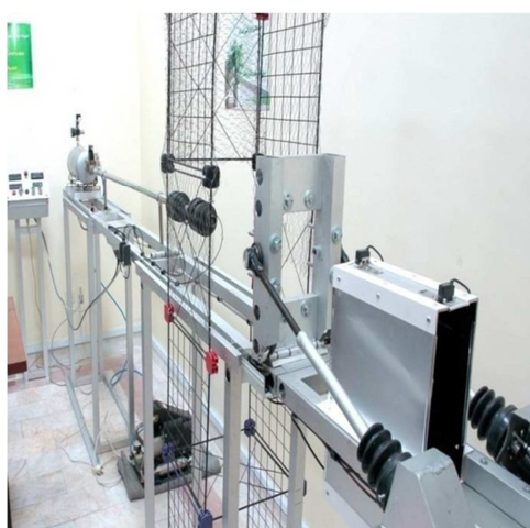
شکل ۳- نمای کلی از دستگاه ضربه سرعت بالای استفاده شده
