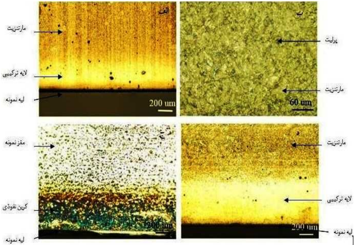
شکل ۴- الف) ریزساختار تشکیل شده در اثر عملیات کربونیتروژن دهی، ب) ریزساختار تشکیل شده در اثر عملیات کربونیتروژن دهی با بزرگنمایی بالاتر، ج) ریزساختار تشکیل شده در اثر عملیات نیتروکربن دهی و د) ریزساختار تشکیل شده در اثر عملیات نیتروژن دهی و سپس کربن دهی
