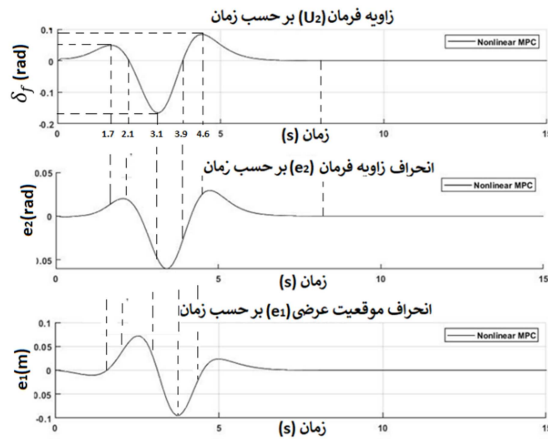
شکل ۵- خروجی زاویه فرمان به همراه انحراف موقعیت عرضی و انحراف زاویه فرمان نسبت به مسیر مطلوب در حین ردیابی مسیر
