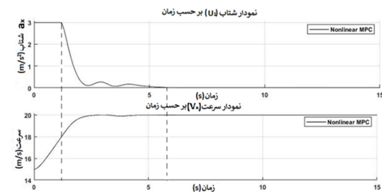
شکل ۴- خروجی نمودار سرعت و شتاب طولی خودرو در حین ردیابی مسیر با روش کنترل غیر خطی مدل پیش بین
