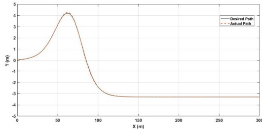
شکل ۳- نتایج شبیه سازی پروفیل تعقیب مسیر خودرو
