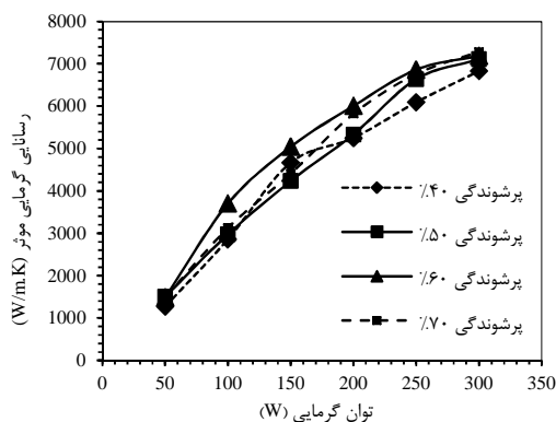
شکل ۵ - نمودار تغییرات رسانایی گرمایی مؤثر به ازای پرشوندگی‌های مختلف در حالت ۹۰ درجه
