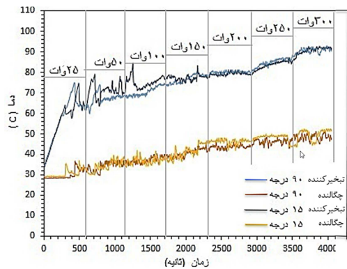
شکل ۱۰- دمای چگالنده و تبخیرکننده در دو زاویه ۹۰ و ۱۵ درجه در توان‌های ورودی مختلف به تبخیرکننده
