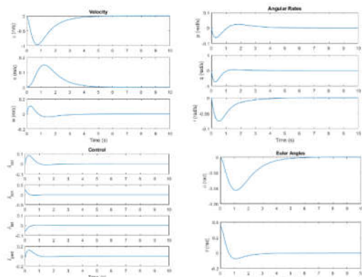
شکل ۷- تاریخچه‌ی متغیرهای حالت و ورودی‌های کنترلی در سرعت ۲۰ نات با بهینه‌سازی و \theta_0 = 20^\circ
