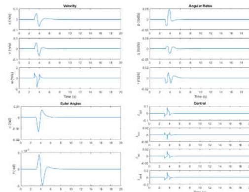
شکل ۹- تاریخچه ی متغیرهای حالت و ورودی های کنترلی در سرعت ۲۰ نات با جایابی قطب و اغتشاش w
