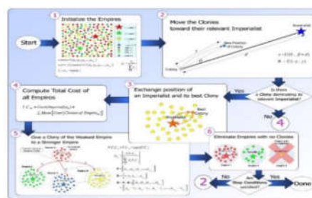
شکل ۱- نمای کلی الگوریتم رقابت استعماری [۱]
