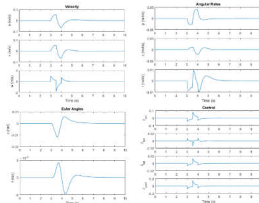
شکل ۱۰- تاریخچه ی متغیرهای حالت و ورودی های کنترلی در سرعت ۲۰ نات با بهینه سازی و اغتشاش w
