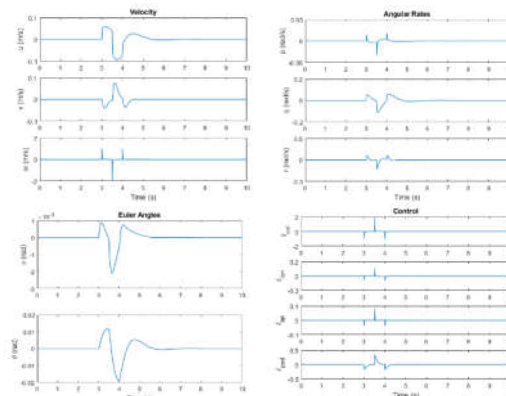
شکل ۱۲- تاریخچه‌ی متغیرهای حالت و ورودی‌های کنترلی در سرعت ۲۰ نات با LQR و اغتشاش w
