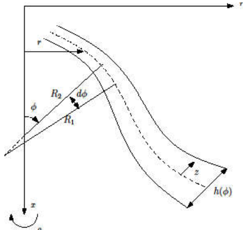
شکل ۱- مقطع پوسته متقارن محوری با انحنای دلخواه
