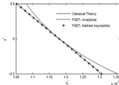
شکل ۳- مقدار حاصل از نظریه کلاسیک و نظریه برشی مرتبه اول
