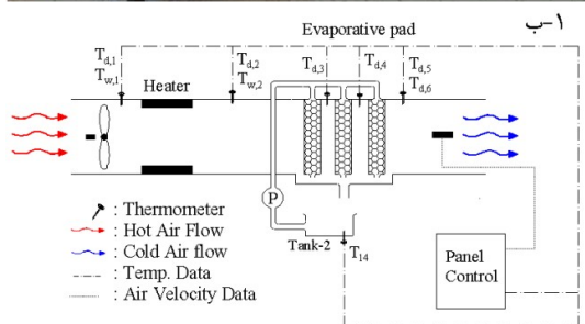
شکل ۱- تصویر (۱-الف) و طرحواره (۱-ب) سیستم سرمایش تبخیری دومرحله‌ای
