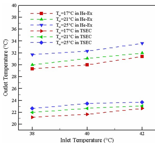
شکل ۶- حساسیت دمای خروجی از سیستم سرمایش تبخیری دومرحله‌ای و مبادله کن نسبت به دمای هوای ورودی در دماهای مختلف آب داخل مبادله کن گرما
