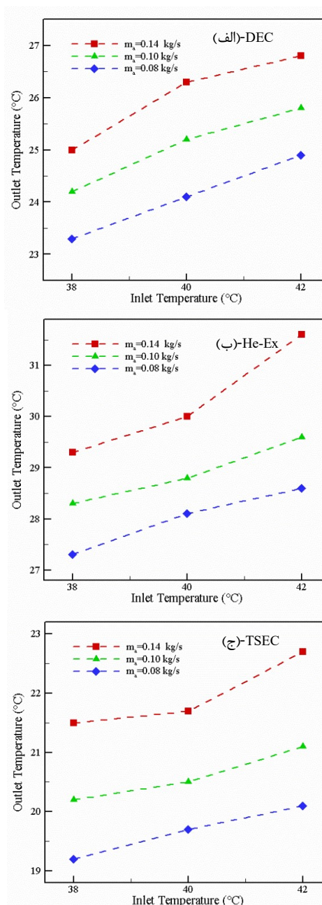
شکل ۶- حساسیت دمای خروجی از سیستم سرمایش تبخیری دومرحله‌ای و اجزاء آن نسبت به دمای هوای ورودی در دبی‌های مختلف هوا
