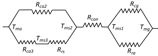
شکل ۳- مدار مقاومت های گرمایی در بازیاب گرمایی تابشی
