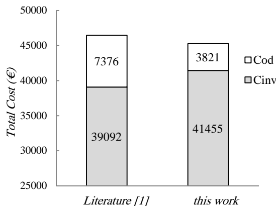
شکل ۷- هزینه های بازیاب گرمایی نمونه سوم
