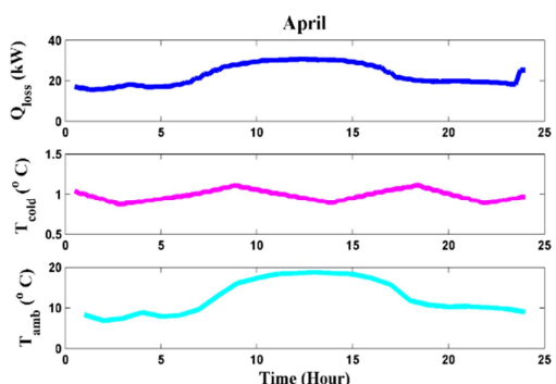
شکل ۶- تغییرات ساعتی بار گرمایی سردخانه، دمای سردخانه، دمای شهر رفسنجان در طول یک روز از ۳ ماه سال به ترتیب (الف) فروردین، (ج) مرداد، (ه) بهمن) برای مبرد R22
