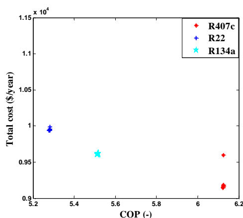
شکل ۳- جبهه‌ی بهینه پارتو برای سه مبرد R407c، R22 و R134a
