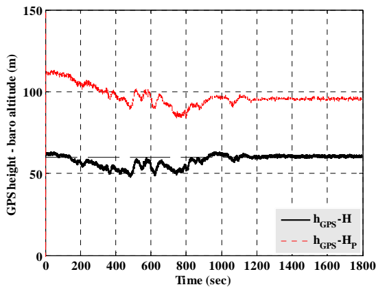
شکل ۵- ارتفاع بارومتری تصحیح یافته و ارتفاع بارومتری سیستم Vitans در مقایسه با ارتفاع GPS
