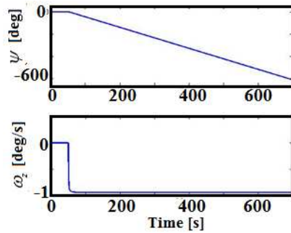
شکل ۷- حرکت زیر دریایی در صفحه افق در طول حرکت زیگ زاگ
