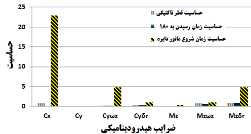
شکل ۸- مقایسه حساسیت ضرایب هیدرودینامیکی در مانور دایره
