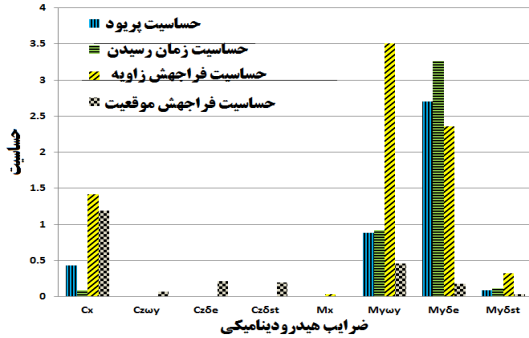
شکل ۱۶- مقایسه حساسیت ضرایب هیدرودینامیکی در مانور زیگ زاگ عمودی
