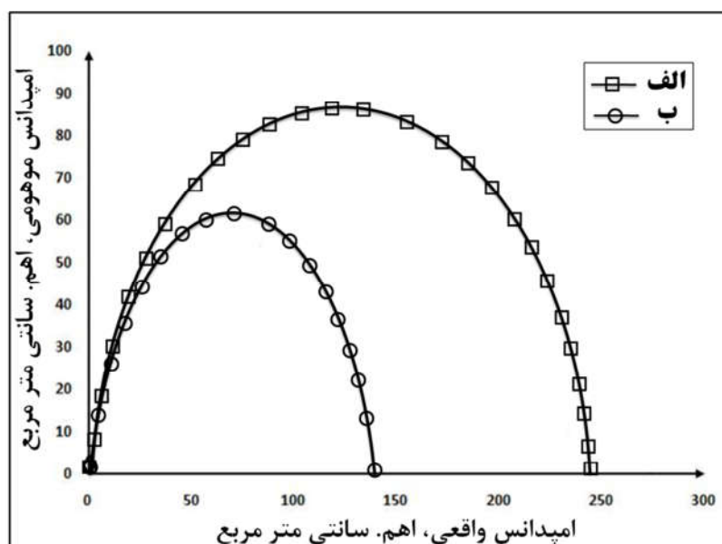
شکل ۵- نمودار نایکویست مربوط به آزمایش طیف سنجی امپدانس الکتروشیمیایی در حداقل سه بار تکرارپذیری: الف) منطقه ذوب اتصال جوشکاری ایجاد شده با ورق‌های حاوی آلومینیوم، ب) منطقه ذوب اتصال جوشکاری ایجاد شده با ورق‌های بدون آلومینیوم
