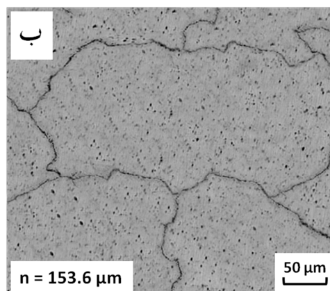
شکل ۲- تصاویر میکروسکوپ نوری در بزرگنمایی ۱۰۰: الف) منطقه ذوب اتصال جوشکاری ایجاد شده با ورق‌های بدون آلومینیوم، ب) منطقه ذوب اتصال جوشکاری ایجاد شده با ورق‌های حاوی آلومینیوم
